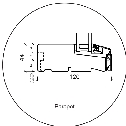
Rama boczna
