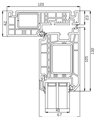
Rama górna
