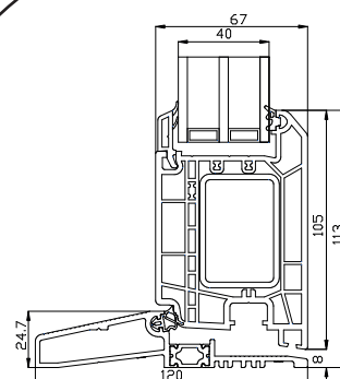
Próg aluminiowy
