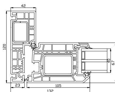
Rama boczna
