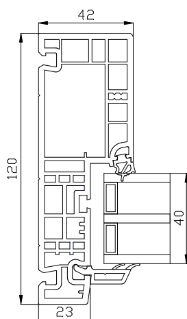
Rama boczna
