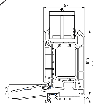
Próg aluminiowy
