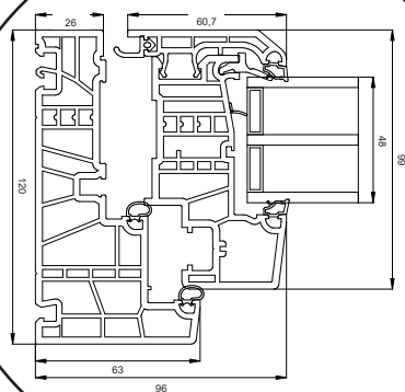
Rama boczna
