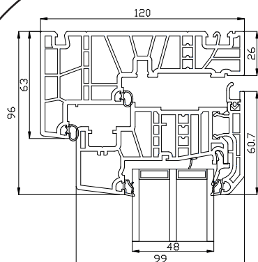
Rama górna
