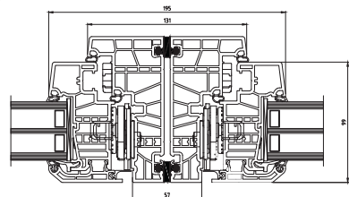
Łączenie pionowe
